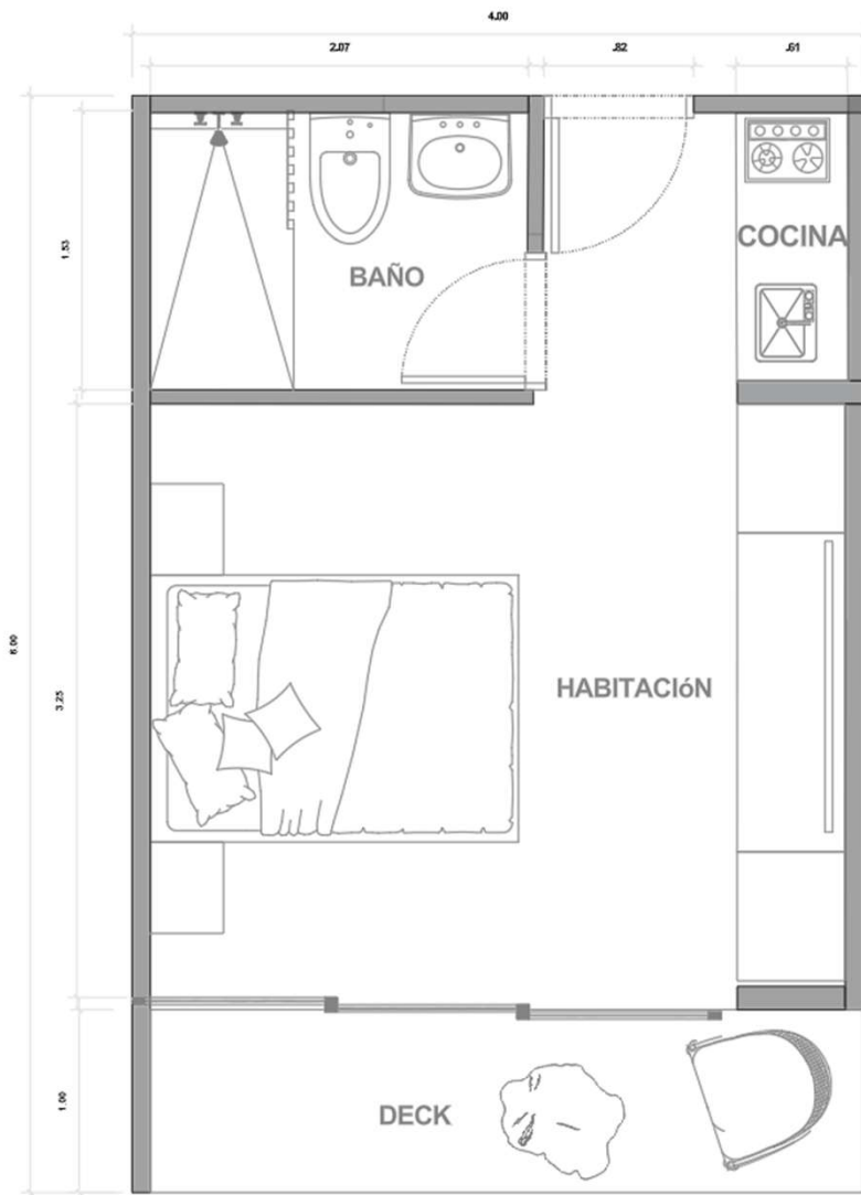
Planta general bungalow – 1 Nivel Escala 1-50
